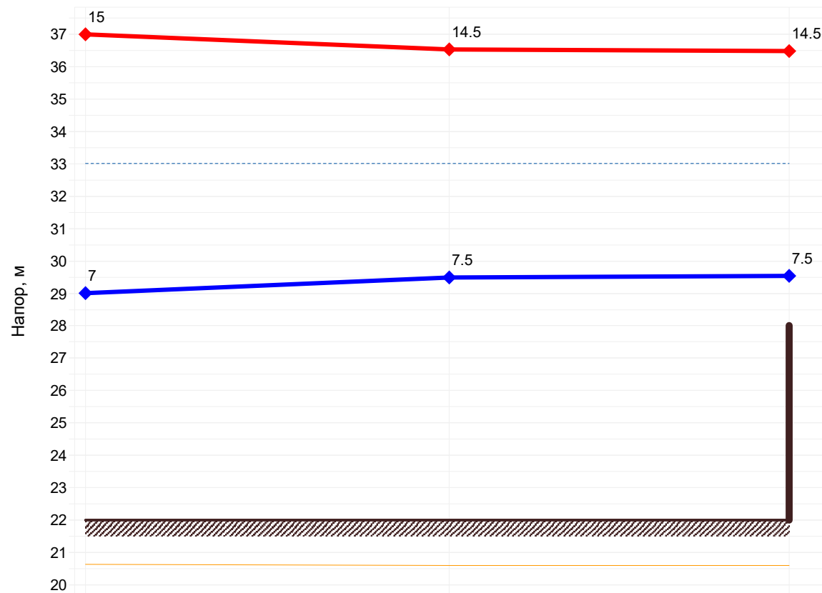
Пьезометрический график от «Кот №58» до «МБОУ СОШ № 4»
